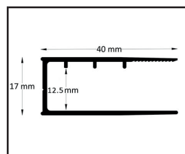
Festes Glaswandprofil
