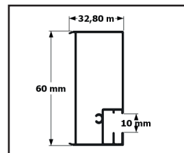
Perfil vetro
