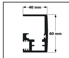
Perfil carril
