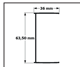
Profil przyścienny
