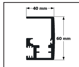
Profil prowadnicy
