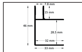
Eckprofil
