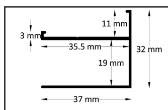
Festes Wandprofil
