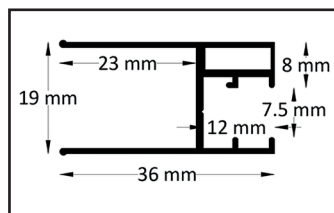
Festes Glasprofil
