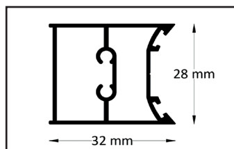
Profil des Scharniers
