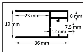
Perfil de cristal fijo
