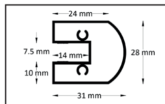
Perfil giratorio de cristal
