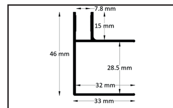
Perfil de esquina
