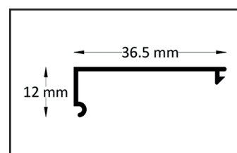
Couverture de profil mural
