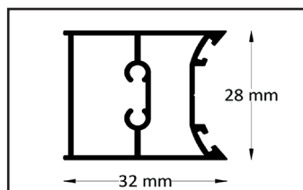
Profilo cerniera
