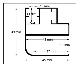
Eckprofil
