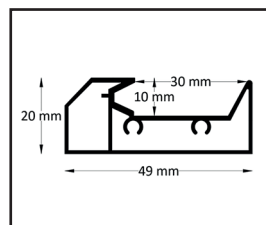
Binäres Profil
