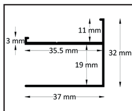
Wandprofil
