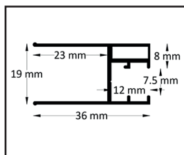
Festes Glasprofil
