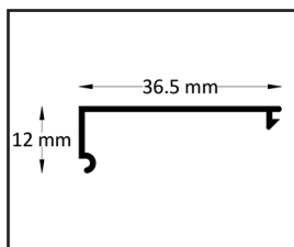
Wandprofilabdeckung
