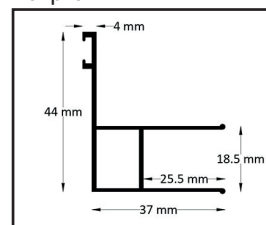
Profil des Türverschlusses
