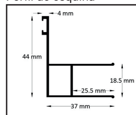
Perfil cierre de la puerta
