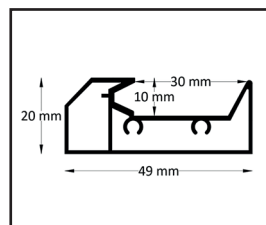
Profil binaire
