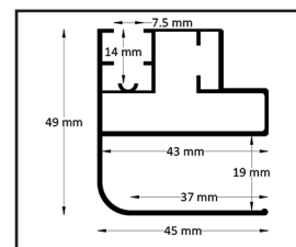
Profilé d'angle
