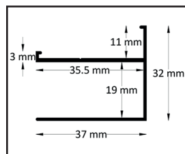
Profilé wall
