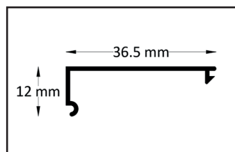
Cover profil de mur
