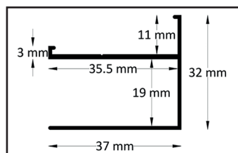
Profil de mur
