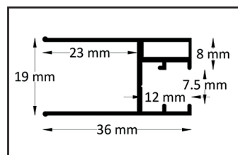
Profilé de verre fixe
