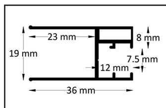
Profil szyby stałej
