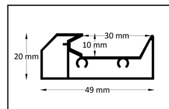
Profilo binario
