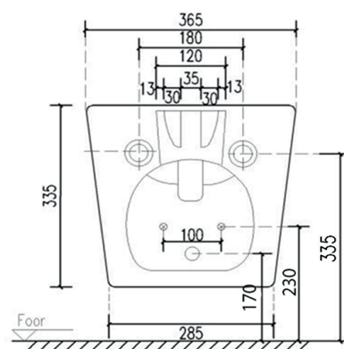
BIDET (art.GIO.25)
