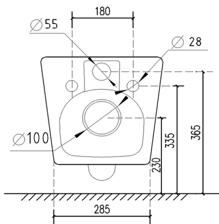
TOILETTE (art.GIO.24)
