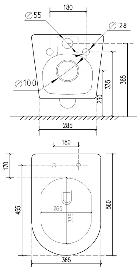
CUVETTE (art.GIO.24)
