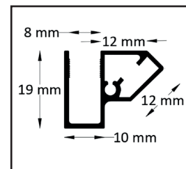
Profilo angolo
