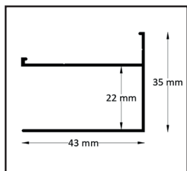
Profilo muro
