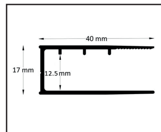
Wandprofil
