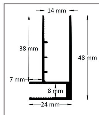
Perfil de esquina
