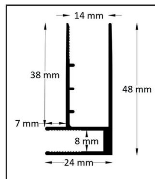
Profilé d'angle
