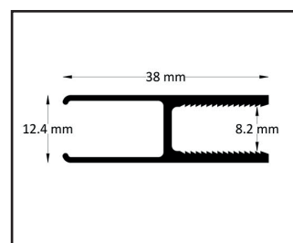
Profil kątowy
