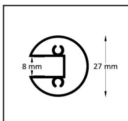
Profilo vetro rotante
