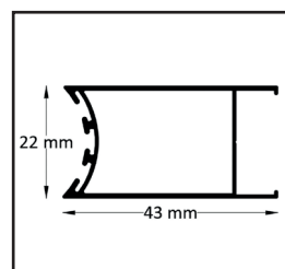
Profil zawiasu
