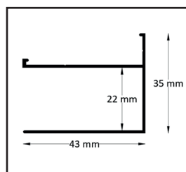
Profil przyścienny
