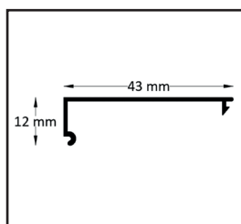
Cubierta perfil muro
