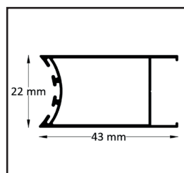
Perfil de bisagra
