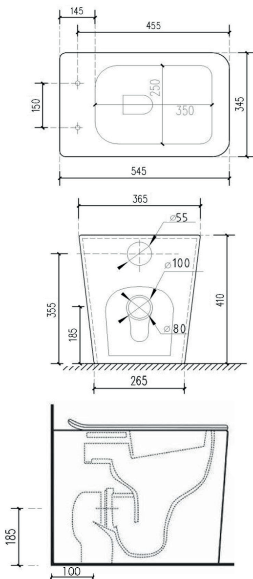
INODORO (art.GIO.22RIM)
