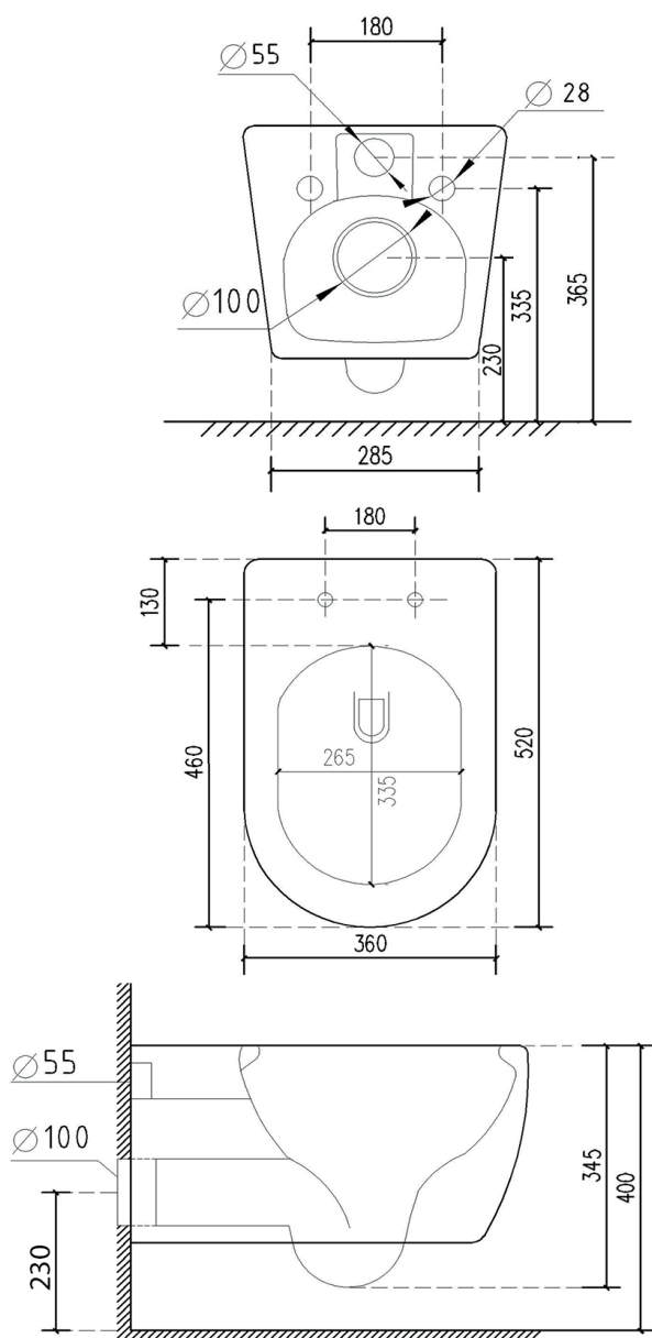
WC (art.GIO.24RIM)
