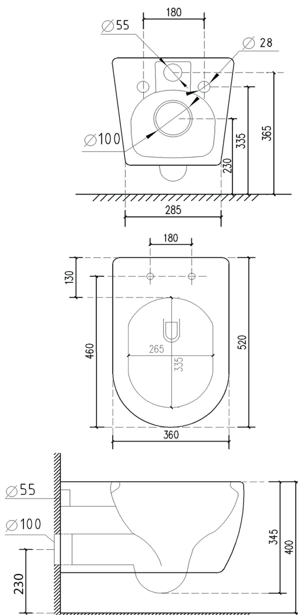
WC (art.GIO.24RIM)
