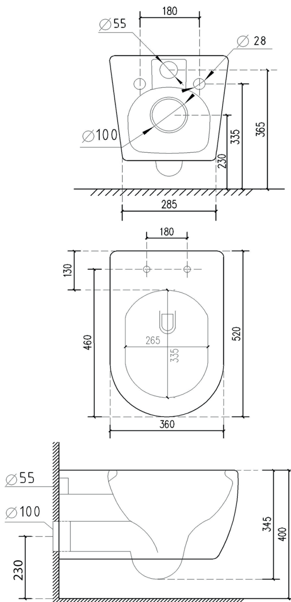
WC (art.GIO.24RIM)
