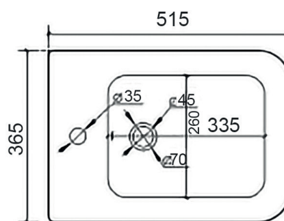
BIDET (art.GIO.31BLACK)
