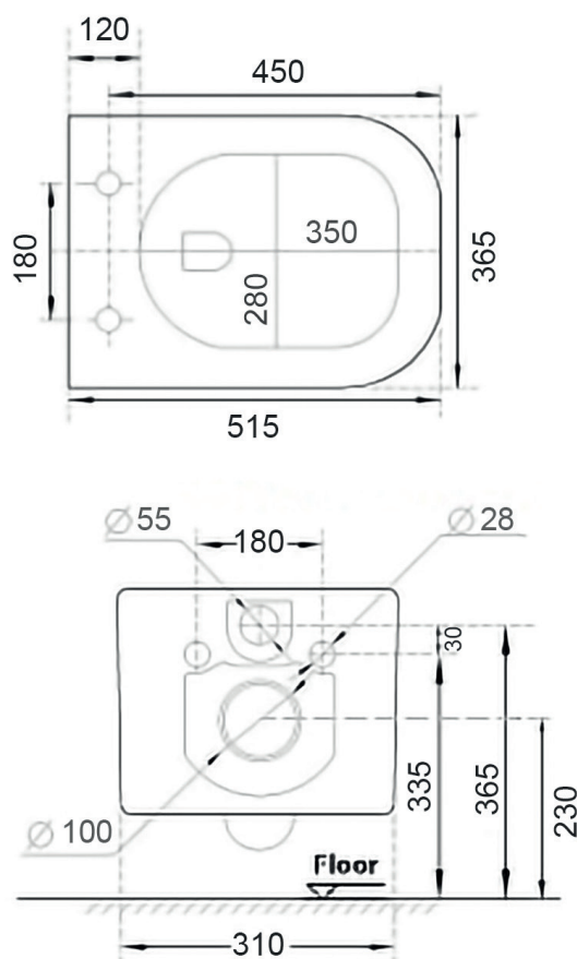
WC (art.GIO.30BLACK)
