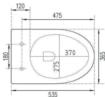
INODORO (art.GIO.40)
