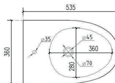
BIDET (art.GIO.41)
