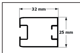
Profil de l'aimant
