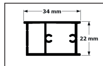
Telaio orizzontale
