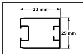
Profil magnetyczny
