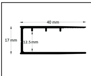
Wandprofil
