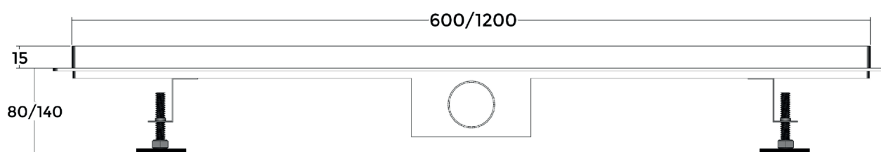
Section longitudinale
