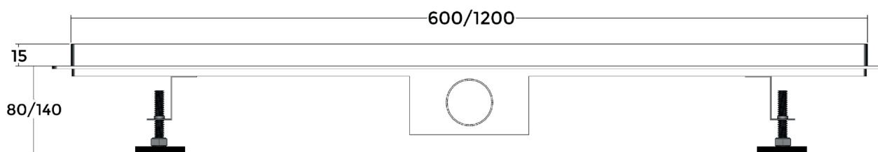
Przekrój podłużny
