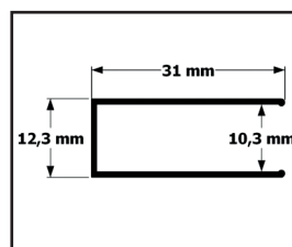
Perfil de la pared lateral
