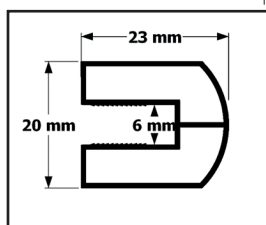
Perfil de vidrio
