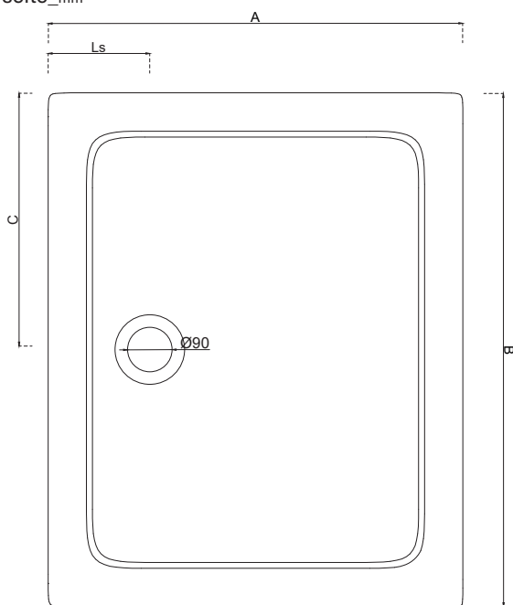
Abschnitt_mm
