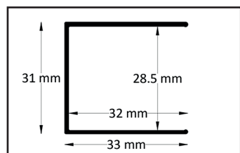
Wandprofil
