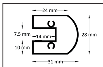
Glas-Drehprofil
