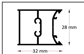
Perfil de bisagra
