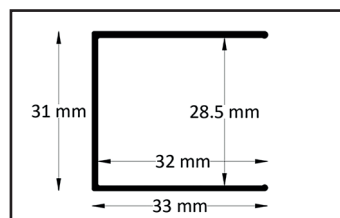
Profilé mural fixe
