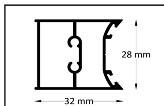
Profil de la charnière
