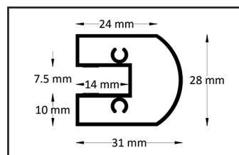
Profilé rotatif en verre
