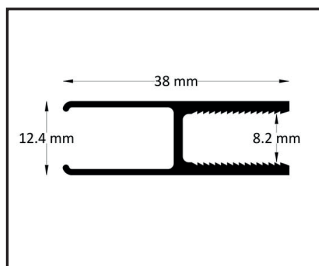
Perfil vetro
