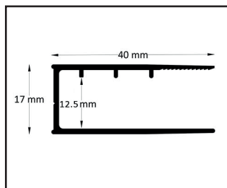
Profil wall
