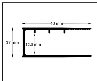
Profil przyścienny
