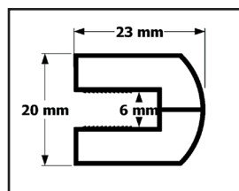
Glasprofil
