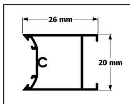
Profil des Scharniers
