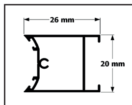
Profil de la charnière
