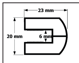
Profilé de verre
