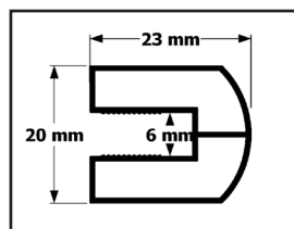
Profilo vetro
