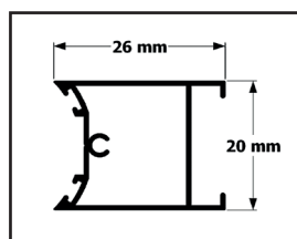
Profil zawiasu
