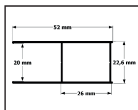
Profil przyścienny
