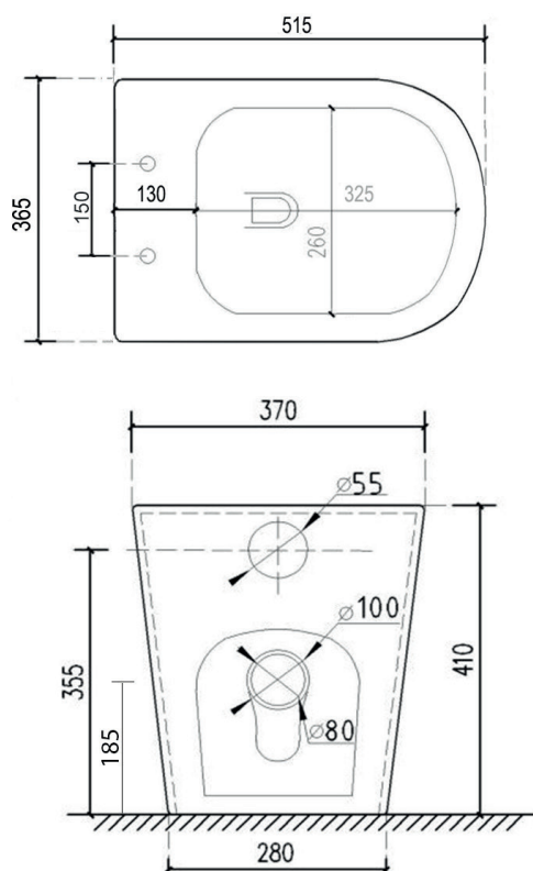
MISA WC (art.GIO.42)
