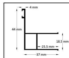
Profil fermeture de porte
